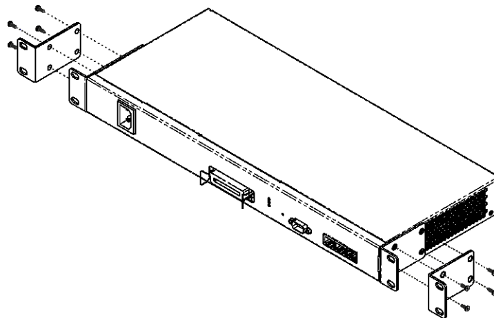
Рисунок 5 – Крепление кронштейнов
